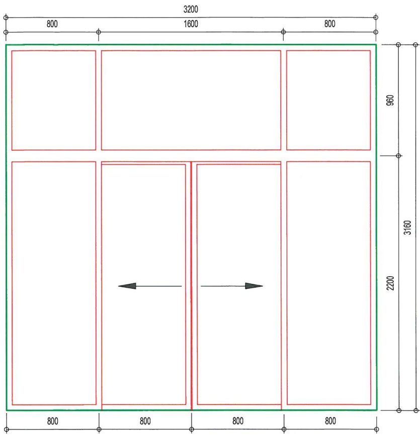
Scianka z drzwiami rozsuwanymi kpl. 1
